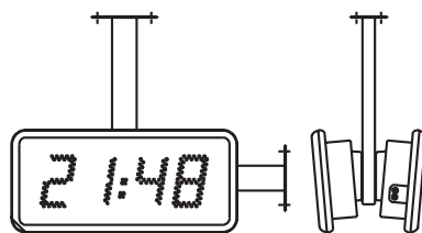
Doppelseitige Wand- oder Deckenmontage
